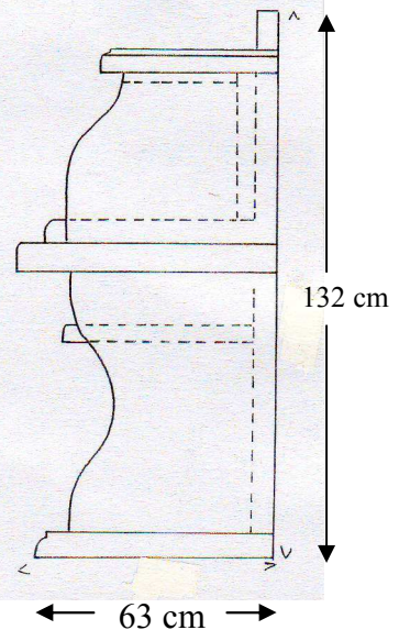
VUE DE PROFIL
