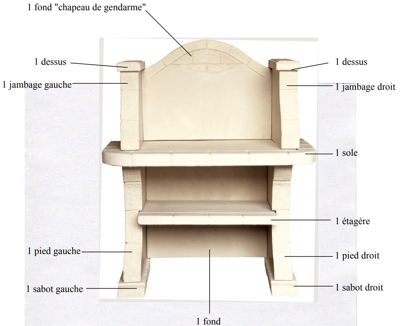
Barbecue composé de 12 pièces
